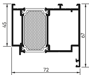
Рама дверна зовнішнього відкриття арт. 72FDT-T
