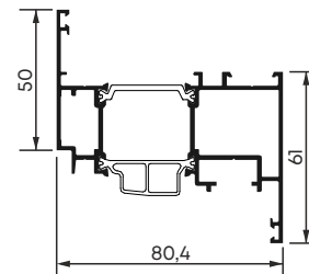
Стулка віконна середня компланарна під ПВХ фурнітуру арт. 72PVW2-C
