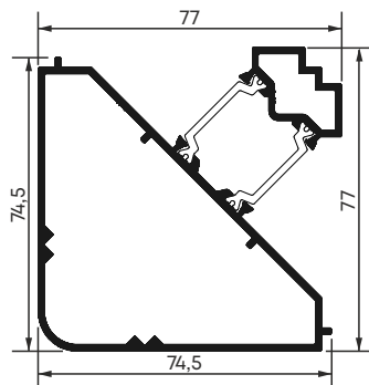
Профіль поворотний арт. 72D02
