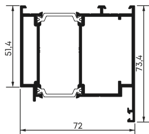
Рама дверна посилена зовнішнього відкриття арт. 72FDT2
