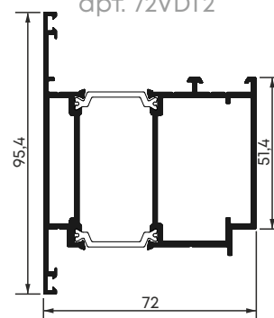
Стулка дверна посилена зовнішнього відкриття арт. 72VDT2
