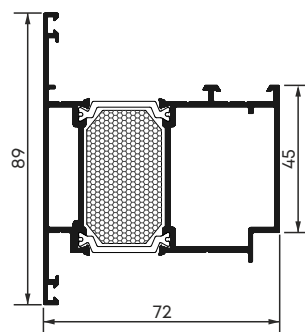
Стулка дверна зовнішнього відкриття арт. 72VDT-T
