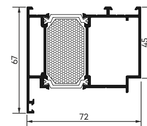
Рама дверна внутрішнього відкриття арт. 72FDZ-T
