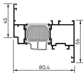
Стулка віконна середня компла- нарна з пазом під фурнітурну тягу арт. 72VW2-C-T
