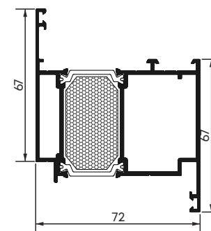
Стулка дверна внутрішнього відкриття арт. 72VDZ-T
